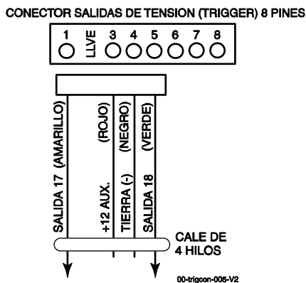
Figura 12. Conector Salidas de Voltaje en Placa (Trigger) con Cable 4 Hilos para Uso solo de Salidas de Voltaje
