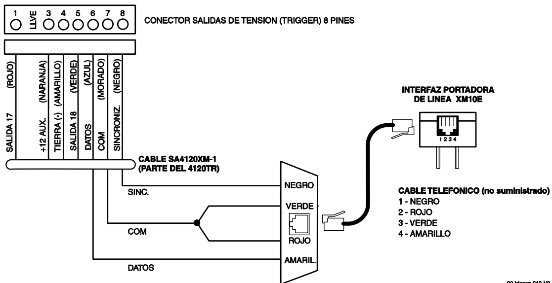
Conexiones Interfaz Portadora de Línea XM10E
