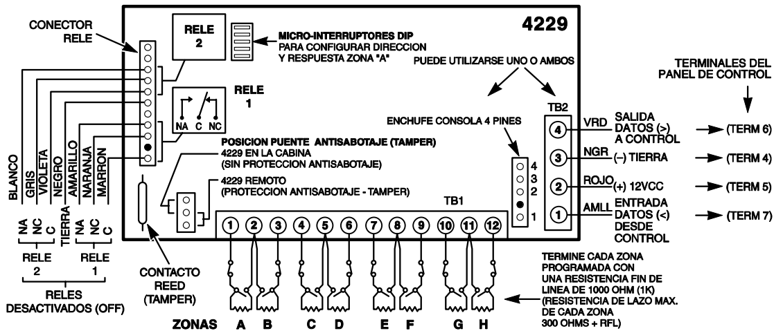
Figura 7. Conexiones 4219 y 4229 (4229 mostrado)
