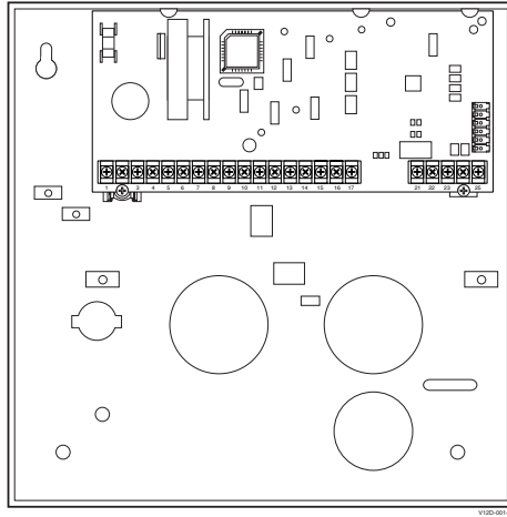
Figura 2. Montaje de la Tarjeta de Circuito Impreso
