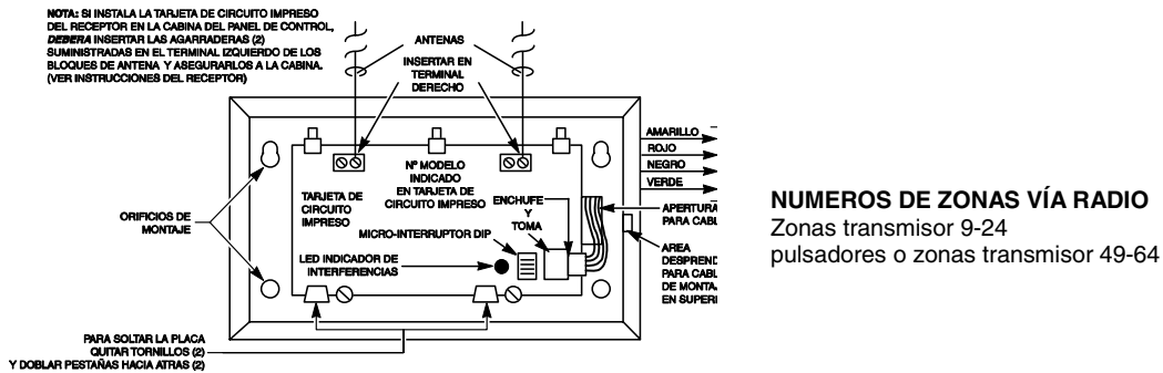
Figura 8. Receptor Vía Radio 5881EN (sin tapa)
