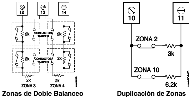
Figura 5. Configuración de Zonas
