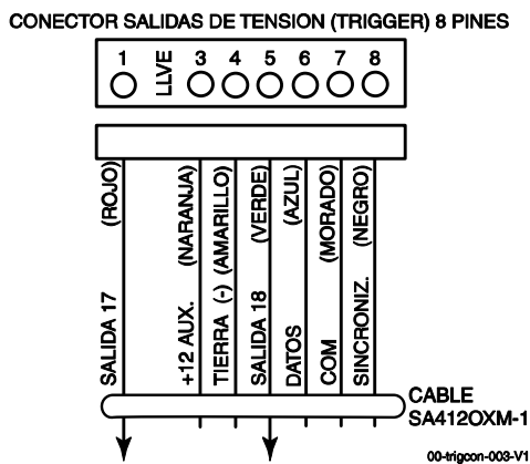
Figura 11. Conector de Salidas de Voltaje en Placa (Trigger) con Cable SA4120XM-1 para Usar con Módulo Interfaz de Portadora de Línea X10
