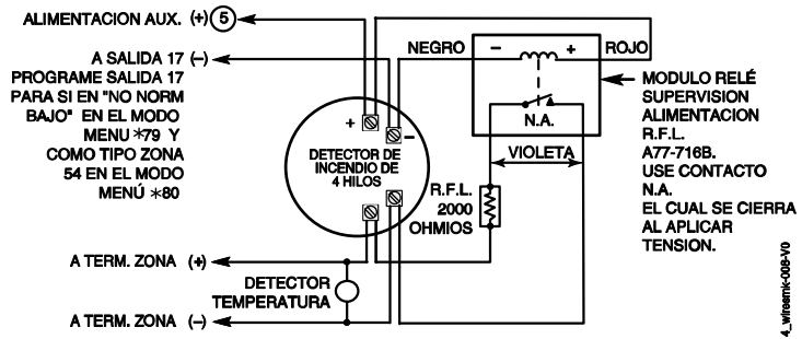
4 Detector de Incendio de 4 Hilos Usando Restablecimiento de Alimentación
