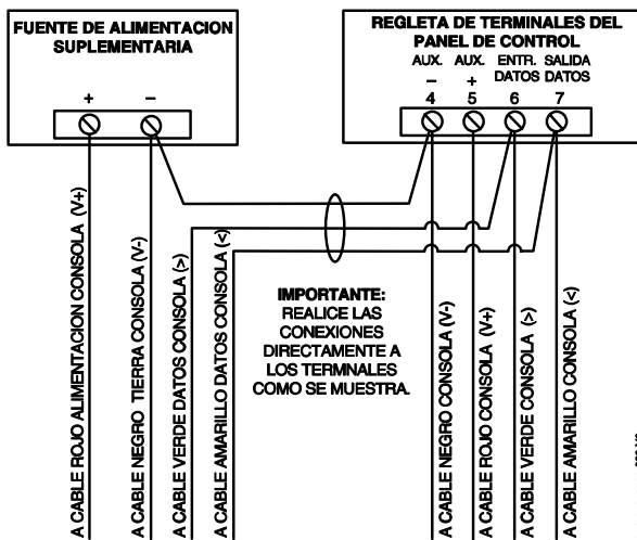
Figura 3. Fuente de Alimentación Suplementaria
