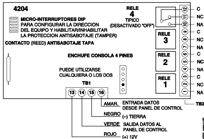
Figura 10. Conexiones del Módulo 4204 al Panel de Control
