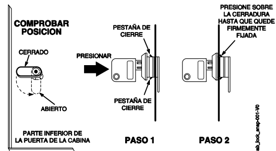
Figura 1. Instalación de la Cerradura de la Cabina
