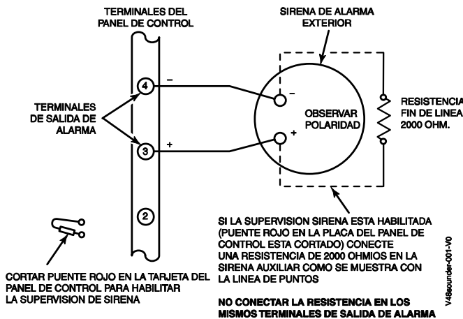
Figura 4. Cableado Sirena (Supervisado)
