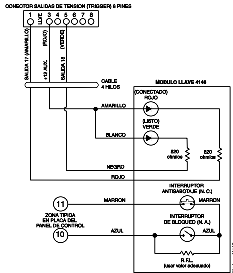
Figura 9. Cableado Módulo Conexión/Desconexión por Llave
