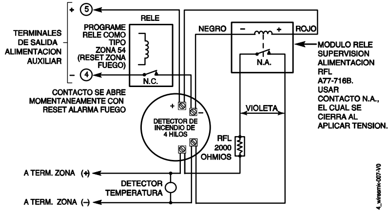
4 Detector de Incendio de 4 hilos usando Relé para Salida 17 para Restablecimiento de Alimentación
