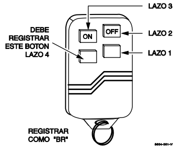
5804 Llave/Transmisor Vía Radio
